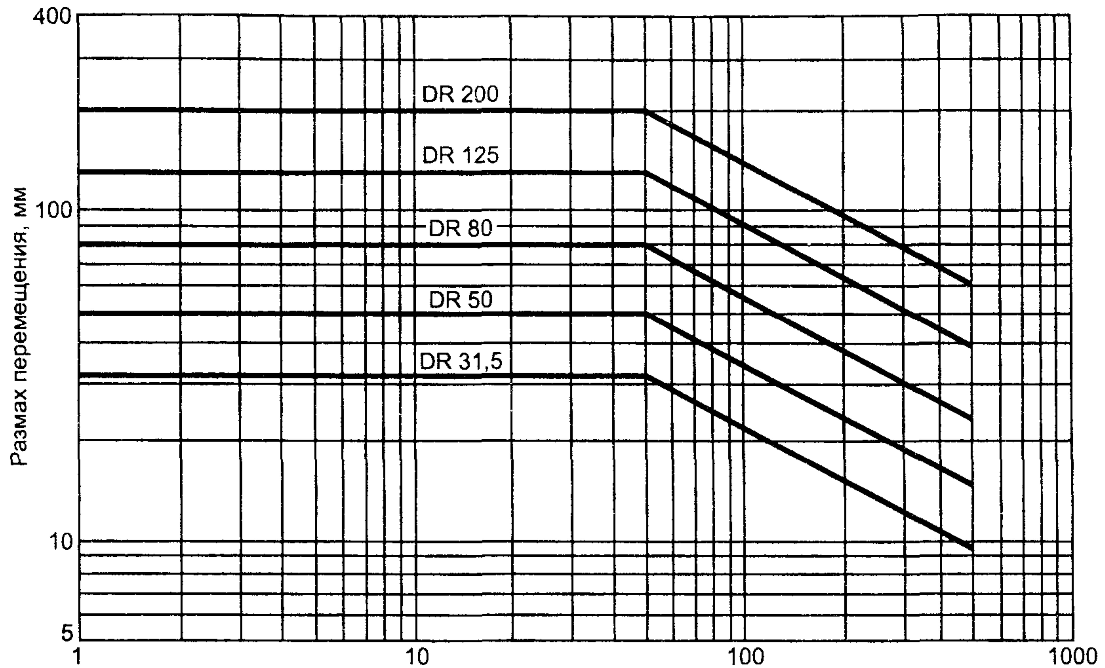
Рисунок 1 — Кривые классов вибрации для вибрации вала
