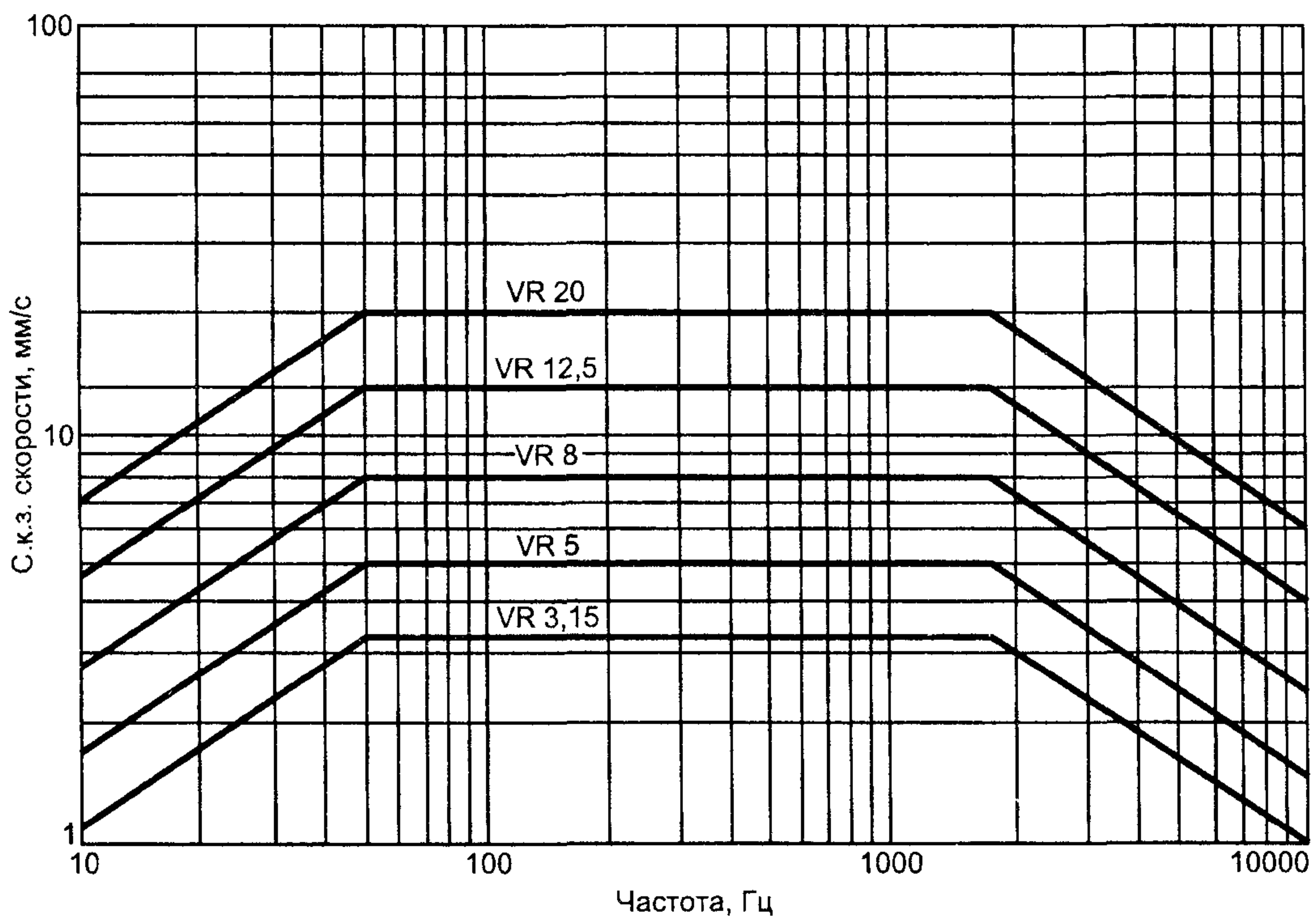
Рисунок 2 — Кривые классов вибрации для вибрации корпуса
